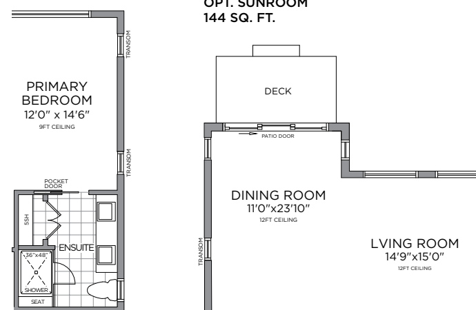
OPT. ENSUITE LAYOUT
